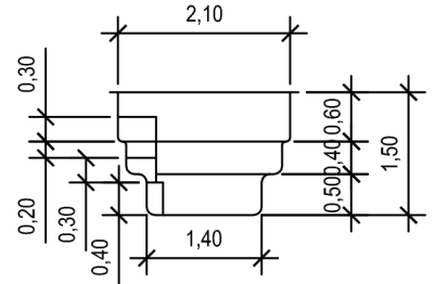
Vue de Coupe/Querschnitt/Sección 3
