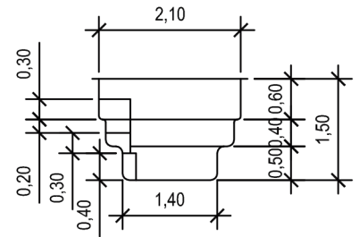
Vue de Coupe/Querschnitt/Sección 3
