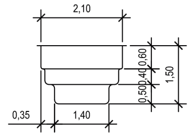
Vue de Coupe/Querschnitt/Sección 1
