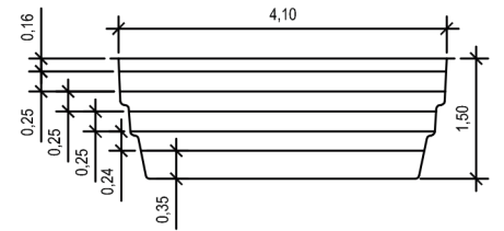
Vue de Coupe/Querschnitt/Sección 3
